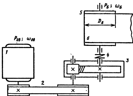
Рис. 12.12. Привод ленточного конвейера с цилиндрическим редуктором и клиноременной передачей:
