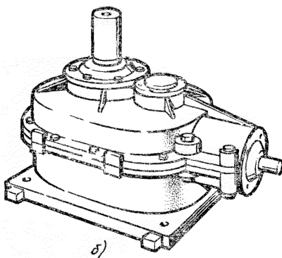
Рис. 2.12. Двухступенчатый коническо-цилиндрический редуктор с вертикальным тихоходным валом: а — кинематическая схема; б — общий вид
