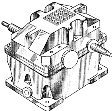
Рис. 10.22. Корпус редуктора с уменьшенным числом выступающих элементов
