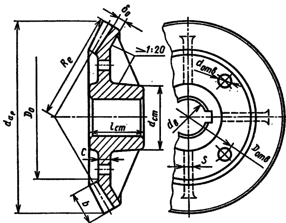
Рис. 10.5. Коническое зубчатое литое колесо при d_{ae} > 300 мм
