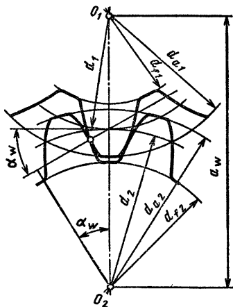
Рис. 3.2. Геометрия зубчатого эвольвентного зацепления
