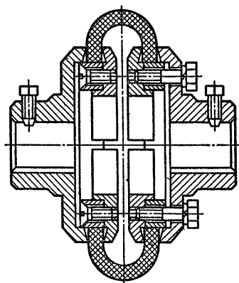
Рис. 11.2. Муфта с торообразной оболочкой
