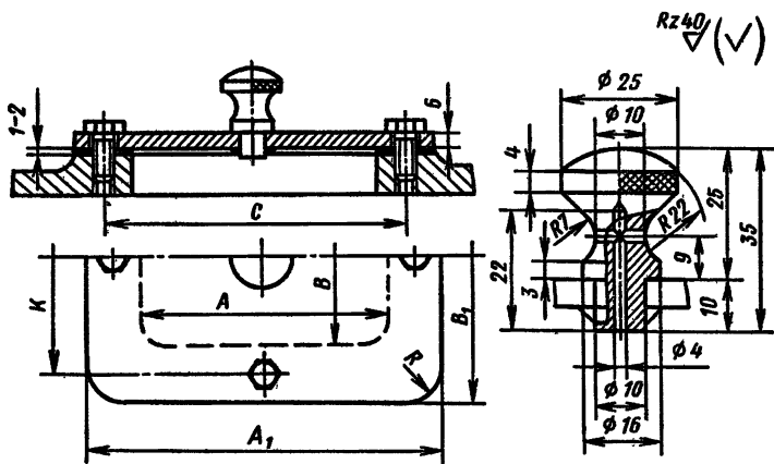
Рис. 10.20. Крышка смотрового отверстия (размеры, мм):
