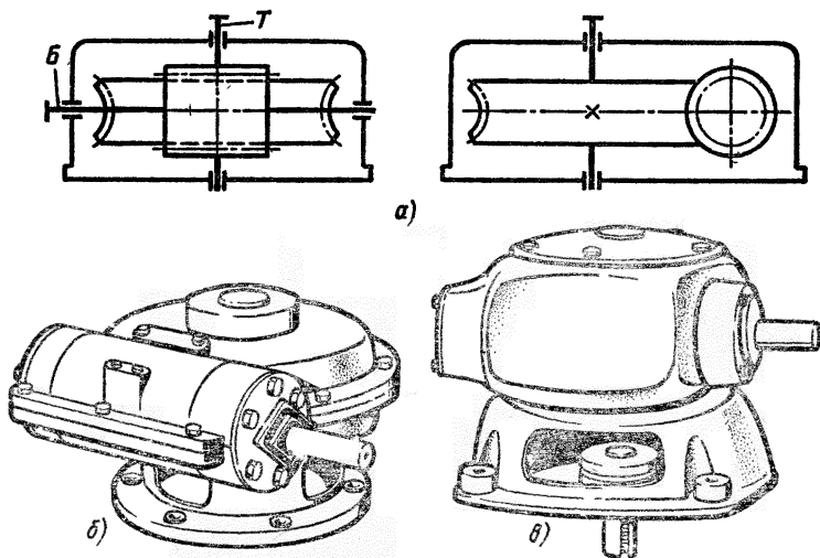
Рис. 2.16. Червячный редуктор с вертикальным валом червячного колеса: a — кинематическая схема; б — общий вид редуктора с разъемным корпусом; в — общий вид редуктора с неразъемным корпусом
