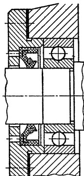
Рис. 9.42. Узел подшипника с магнетным уплотнением (закрытые)
