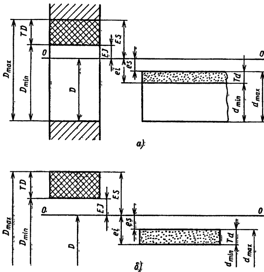
Рис. 10.41. Поля допусков отверстия и вала:
