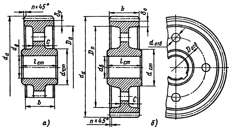
Рис. 10.2. Цилиндрические зубчатые колеса при d_a < 500 мм: а — кованные; б и в — штампованные; з — заготовка, полученная штамповкой в двухстороннем штампе
