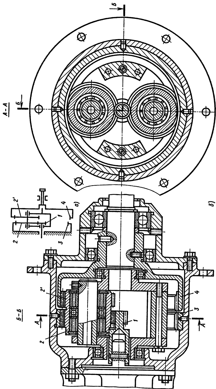
Рис. 5.18. Планетарный редуктор по схеме 5 табл. 5.1 с жестко установленными центральными колесами: a — кинематическая схема; б — общий вид
