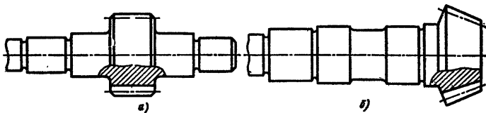
Рис. 10.6. Вали-шестерни: а — цилиндрическая шестерня; б — коническая
