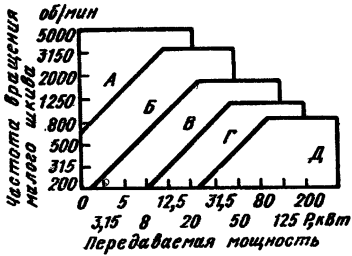
Рис. 7.3. Номограмма для выбора сечения клинового ремня
