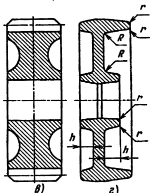
Рис. 10.2. Цилиндрические зубчатые колеса при d_a < 500 мм: а — кованные; б и в — штампованные; з — заготовка, полученная штамповкой в двухстороннем штампе
