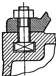
Рис. 10.29. Крепление сборочной единицы к плите болтами.
