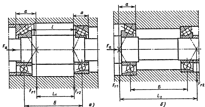
Рис. 9.20. Установка двух радиально-упорных подшипников, поставленных: а – враспор; б – встряжку
