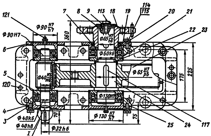
Рис. 12.11. Цилиндрический одноступенчатый зубчатый редуктор
