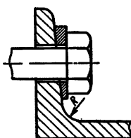
Рис. 10.26. Установка косо́й шайбы
