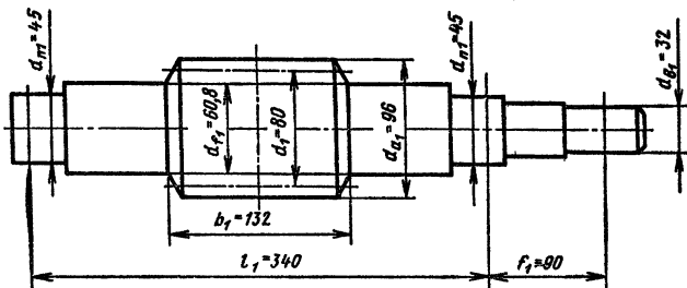
Рис. 12.22. Червяк
