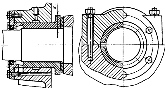
Рис. 9.54. Подшипник для радиальной и осевой нагрузок
