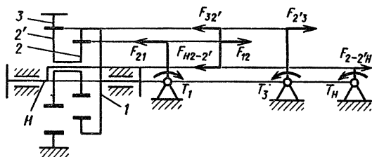
Рис. 5.13. Силовой расчет передачи по схеме 3 табл. 5.1:
