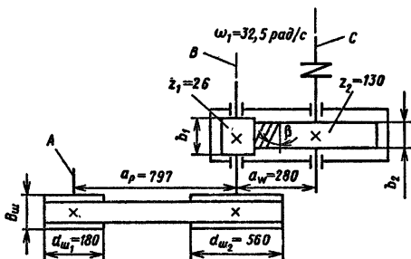
Рис. 12.13. Кинематическая схема привода:
