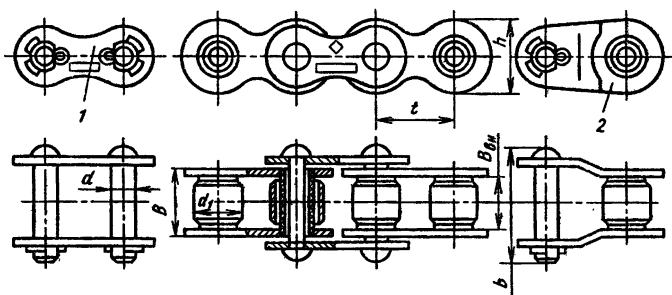
Рис. 7.8. Цепь роликовая однорядная: 1 — соединительное звено; 2 — переходное звено
