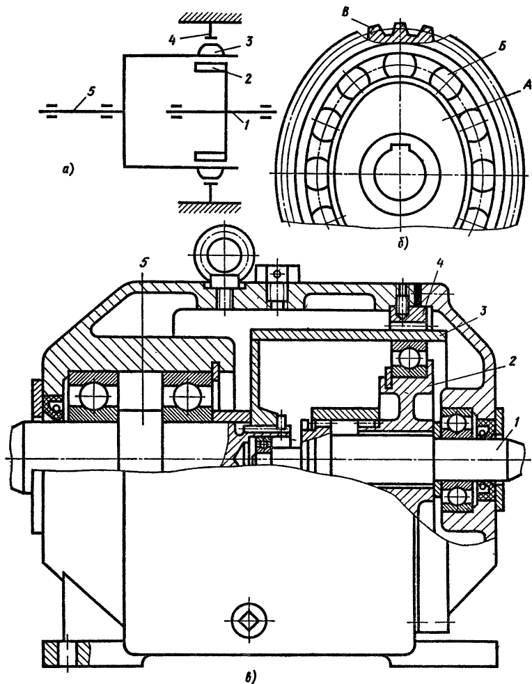
Рис. 2.21. Волновой зубчатый одноступенчатый редуктор: a – кинематическая схема; б – генератор волн; в – продольный разрез
