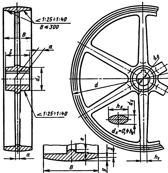
Рис. 7.2. Шків плоскоременної передачі
