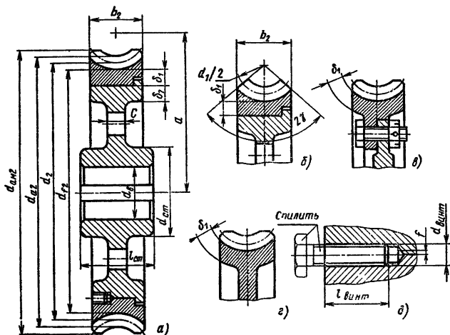
Рис. 10.9. Червячные колеса:
