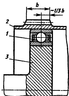
Рис. 6.9. Конструкция кулачкового генератора: 1 — гибкий подшипник; 2 — гибкое колесо; 3 — кулачок
