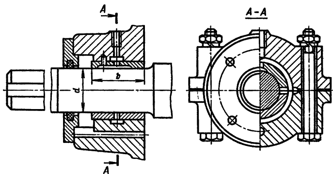
Рис. 9.52. Подшипник скольжения для радиальной нагрузки (без осевой фиксации вала)
