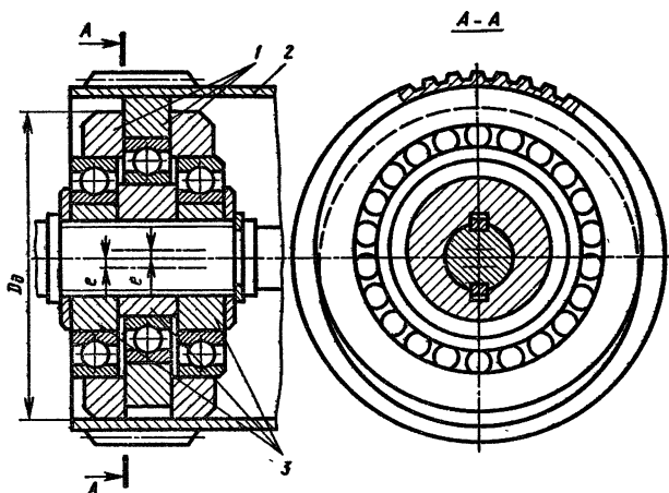
Рис. 6.11. Конструкция дискового генератора без подкладного кольца. 1 – диск; 2 – гибкое колесо; 3 – эксцентрисные втулки
