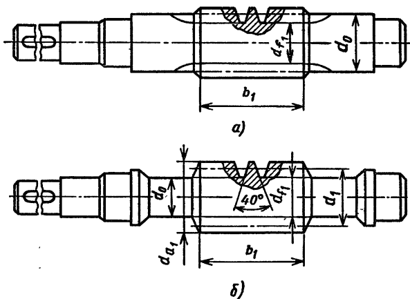
Рис. 10.8. Червяки:
