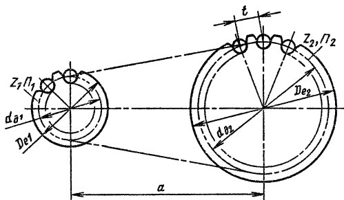
Рис. 7.10. Схема цепной передачи
