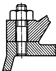
Рис. 10.29. Крепление сборочной единицы к плите болтами.
