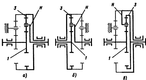
Рис. 5.5. Кинематические схемы планетарных замкнутых дифференциальных передач. Замыкающая передача соединяет:
