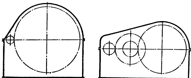
Рис. 2.3. Сопоставление габаритов одноступенчатого и двухступенчатого редукторов с цилиндрическими колесами при одинаковом передаточном числе i = 8,5
