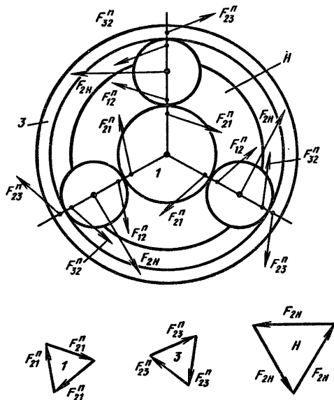
Рис. 5.11. Взаимное уравновешивание сил, действующих в многопоточных передачах
