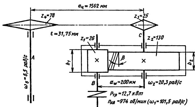
Рис. 12.2. Кинематическая схема привода:
