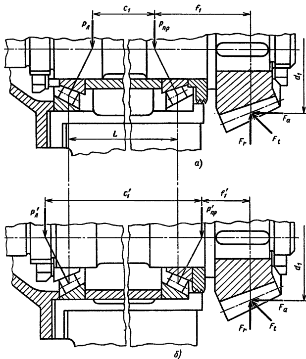
Рис. 12.20. Установка вала конической шестерни на радиально-упорных подшипниках:
