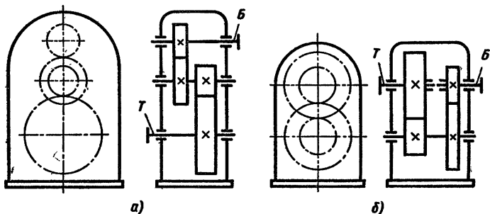
Рис 2.10. Кинематические схемы двухступенчатых цилиндрических вертикальных редукторов:
