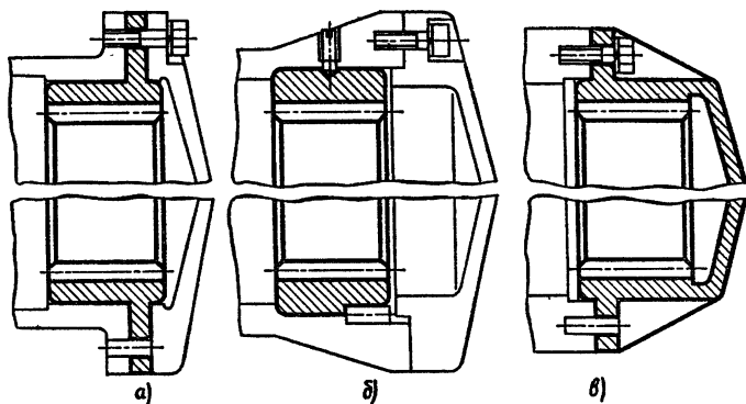
Рис. 5.19. Жесткая установка корончатых колес:
