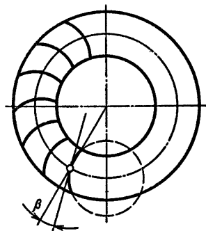
Рис. 3.5. Схема конического колеса с круговыми зубьями
