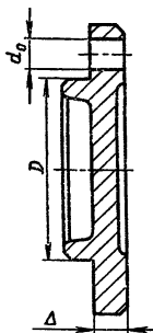
Рис. 12.7. Толщина фланца крышки подшипника:
