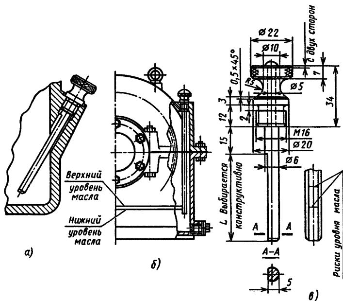
Рис. 10.34. Жезловый маслоуказатель:
