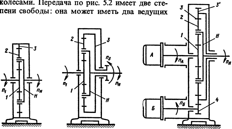
Рис. 5.1. Кинематическая схема планетарной передачи с одной степенью свободы
