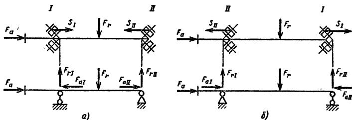
Рис. 9.50. Схема действия сил в радиально-упорных подшипниках, установленных: а — враспор; б — враспяжку
