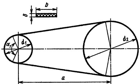
Рис. 7.1. Схема ременной передачи
