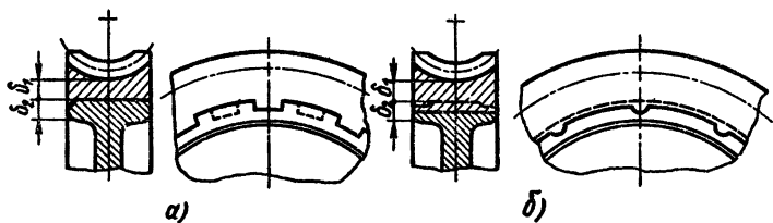
Рис. 10.10. Венцы, отлитые на чугуных центрах:
