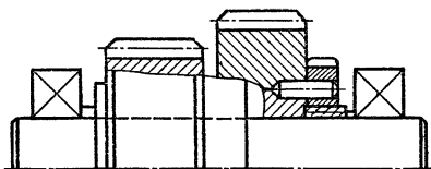
Рис. 5.22. Сборная конструкция сателлитов с двумя венцами с регулировкой их относительного расположения
