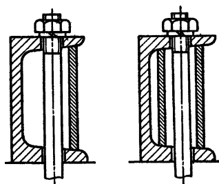
Рис. 10.25. Литая установочная плита
