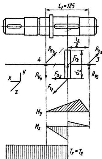
Рис. 12.26. Расчетная схема вала червячного колеса
