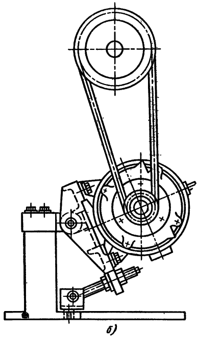
Рис. 7.4. Способы регулирования натяжения ремней установкой электродвигателя: а — на салазках; б — на шарнирной плите
