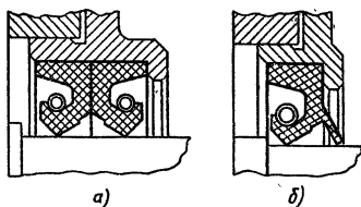
Рис. 9.43. Способы установки магнетных уплотнений
