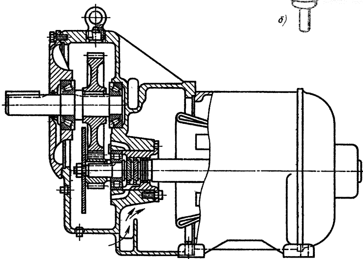
Рис. 2.23. Мотор-редуктор с одноступенчатой зубчатой цилиндрической передачей
