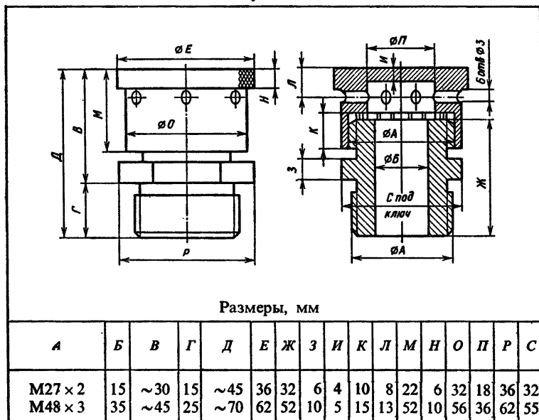
10.6. Отдушина с сеткой
