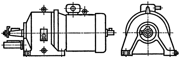
Рис. 5.6. Чертеж мотор-редуктора в исполнении «на лавах»
