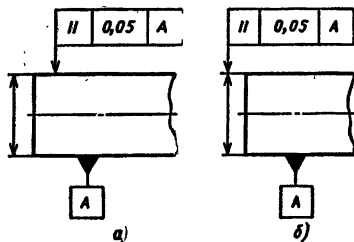
Рис. 10.46. Обозначение допуска по отношению к поверхности и по отношению к оси симметрии: a — допуск по отношению к поверхности; б — допуск по отношению к оси симметрии
