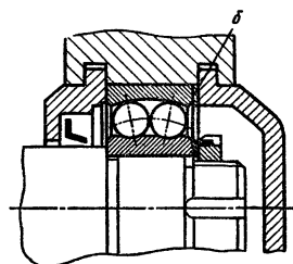
Рис. 9.25. Крепление подшипника между двумя врезными крышками
