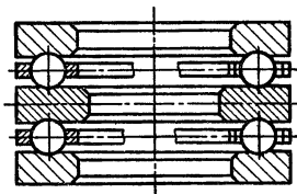
Рис. 9.8. Подшипник шариковый упорный (двухрядный)
