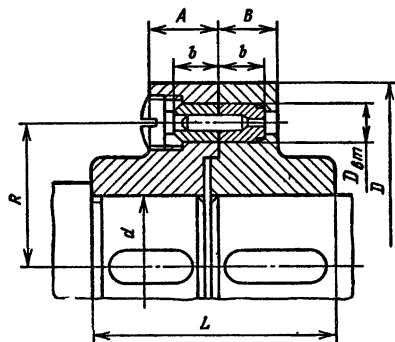
Рис. 11.3. Муфта со срезным штифтом
