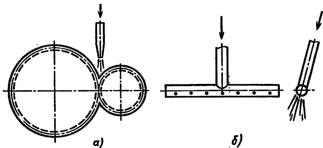
Рис. 10.33. Циркуляционное смазывание
