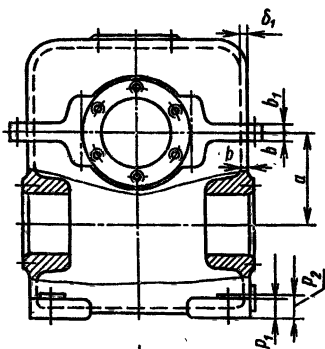
Рис. 10.15. Литые корпус и крышка двухступенчатого цилиндрического редуктора с разъемом по осям валов
