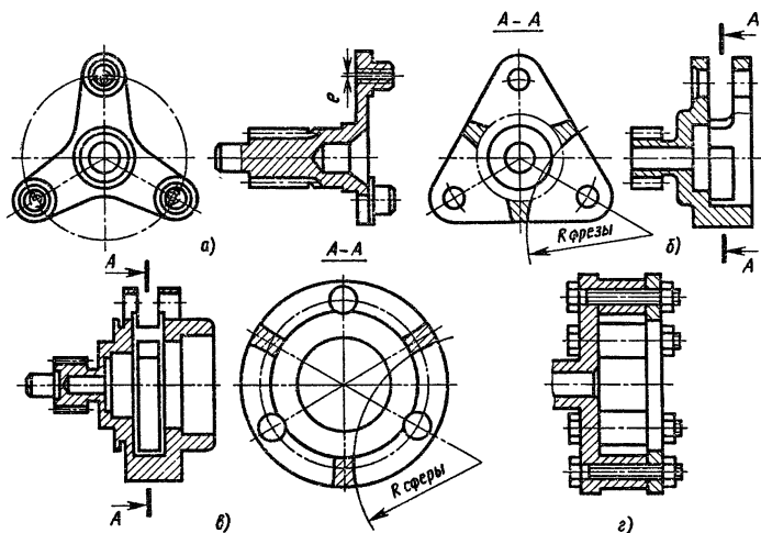
Рис. 5.23. Конструкции водил:
