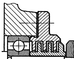
Рис. 9.44. Лабиринтное (осевое) уплотнение
