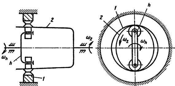
Рис. 6.1. Волновая передача
