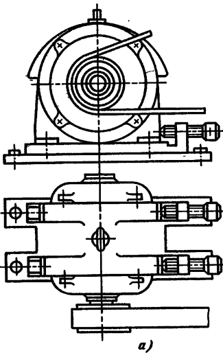
Рис. 7.4. Способы регулирования натяжения ремней установкой электродвигателя: а — на салазках; б — на шарнирной плите
