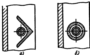
Рис. 10.28. Увеличение жесткости полок швеллера
