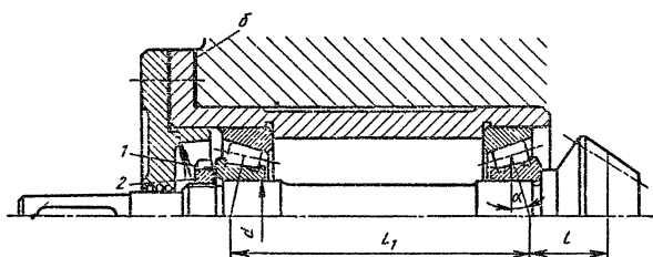
Рис. 9.21. Вал-шестерня на конических роликоподшипниках, поставленных встряжку
