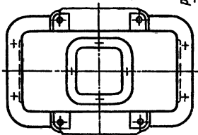
Рис. 10.17. Основание корпуса и крышка червячного редуктора
