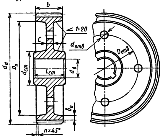
Рис. 10.3. Цилиндрическое зубчатое литое колесо при d_a < 600 мм
