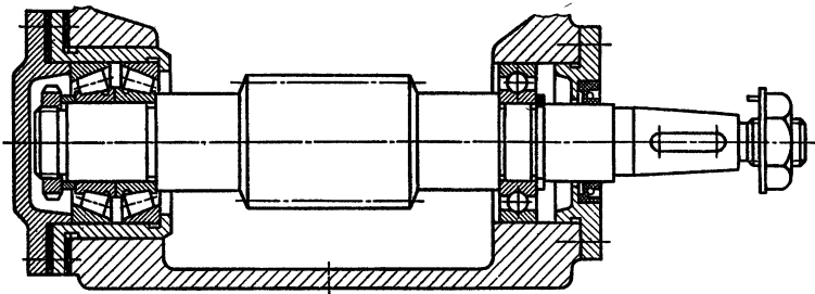
Рис. 9.13. Червячный вал установлен на двух конических роликоподшипниках; правый подшипник – «плавающий» (радиальный однорядный)
