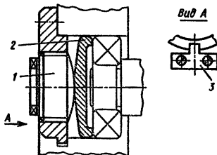
Рис. 9.26. Способ крепления и регулировки радиально-упорного подшипника
