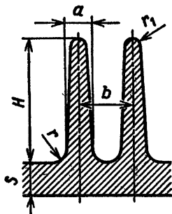
Рис. 10.39. Профиль охлаждающих ребер:
