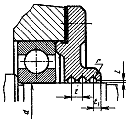
Рис. 9.46. Щелевое уплотнение
