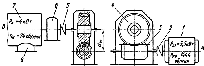
Рис. 12.21. Привод винтового конвейера с червячным редуктором:
