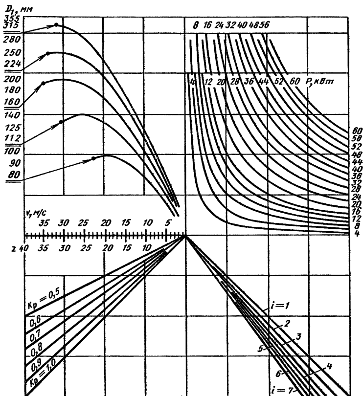
Рис. 7.6. Номограмма для определения числа клиньев полуклинового ремня сечением Л
