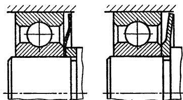
Рис. 9.38. Подшипники с маслоотражательными кольцами
