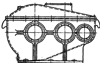
Рис. 10.16. Цельнолитой корпус зубчатого цилиндрического редуктора без разъема
