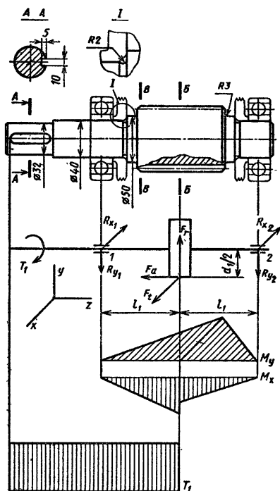
Рис. 12.8. Расчетная схема ведущего вала
