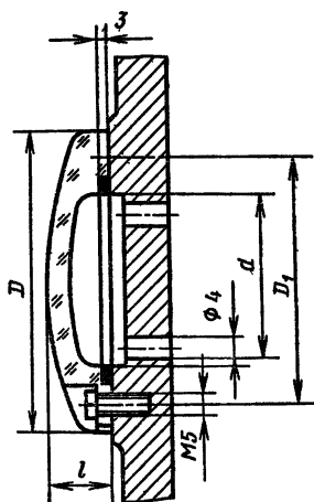
Рис. 10.36. Фонарный маслоуказатель (размеры, мм):
