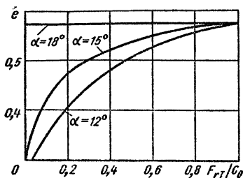
Рис. 9.49. График для определения e в зависимости от F_r/C_0 и \alpha
